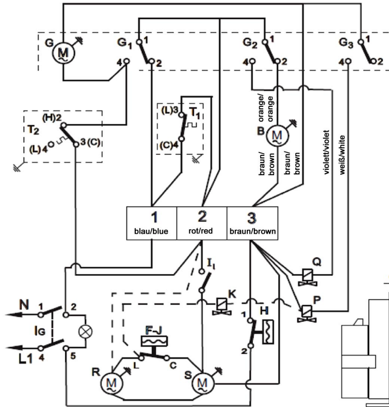
Zeitschaltuhr / timer
